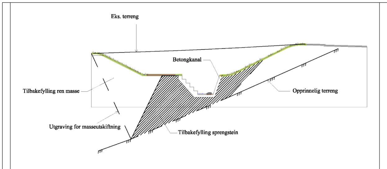
Figur 35. Prinsippskisse av kanalkonstruksjon med masseutskifting av forurensede masser/deponi.
